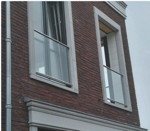
Model Appelscha: gelaagd gehard glas tussen RVS profielen.
